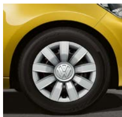
Jante oțel 5 Jx14 cu capace decorative anvelope 165/70 R14 pentru 75 CP Take anvelope 175/65 R14 pentru Move și 60 CP Take
